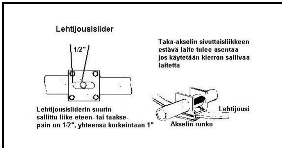
Kuva 7: Lehtijousisliderin asennus
