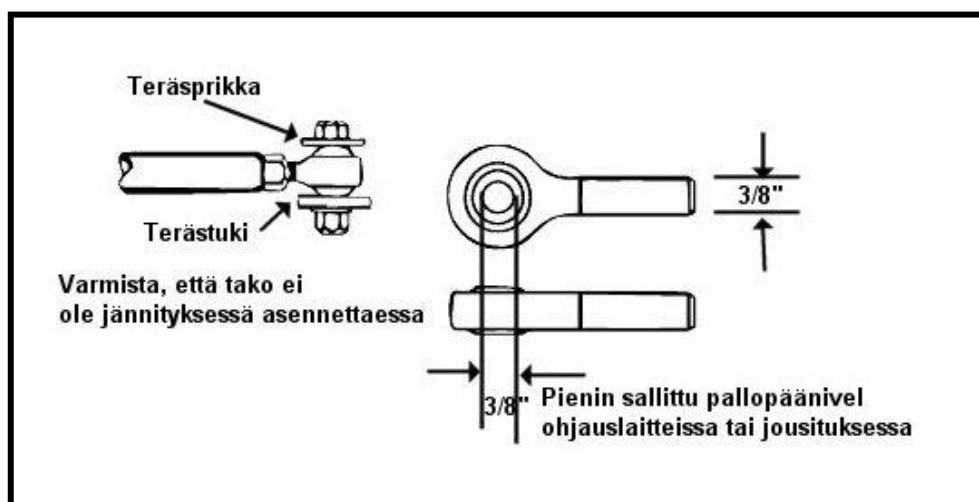
Kuva 8: Pallopäänivelen kiinnitys
