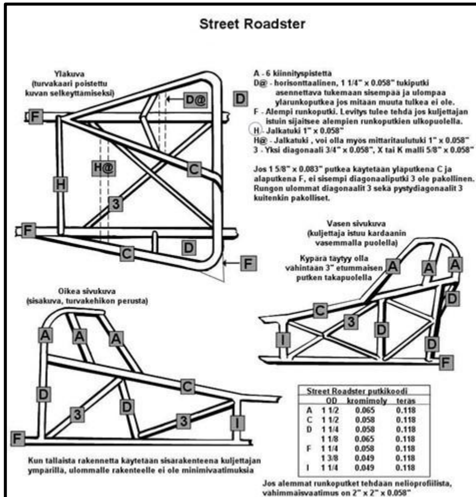
Kuva 17: Street Roadster
