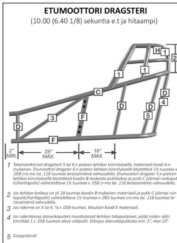
Kuva 14: Etumoottori dragsteri
