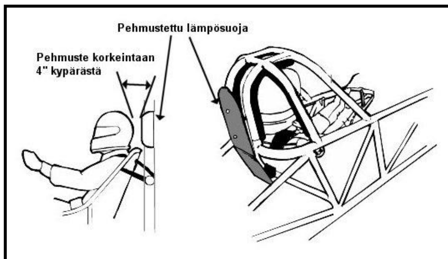
Kuva 24: Pään suojus
