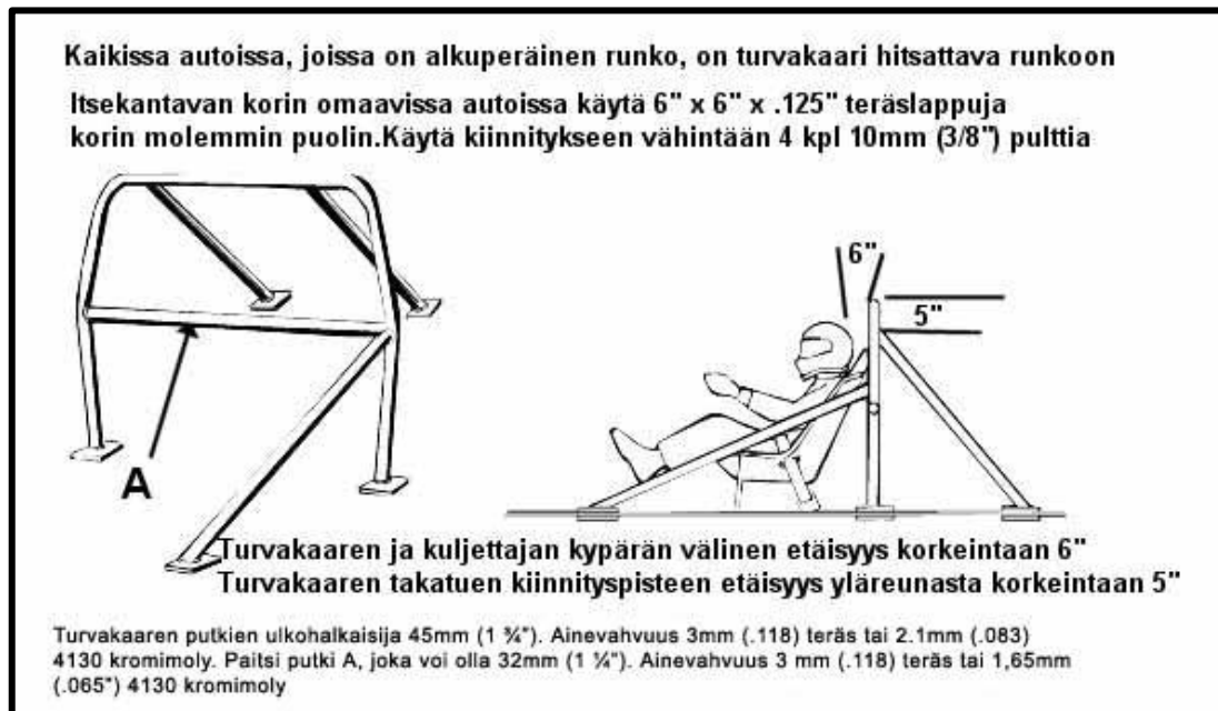
Kuva 13: Turvakaari
