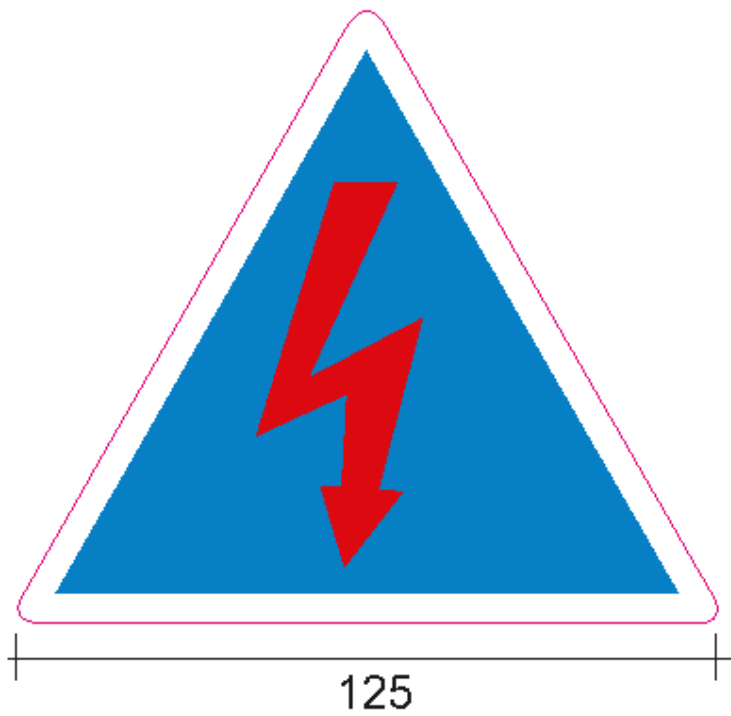
Kuva 30: Päävirtakatkaisin -tarra
