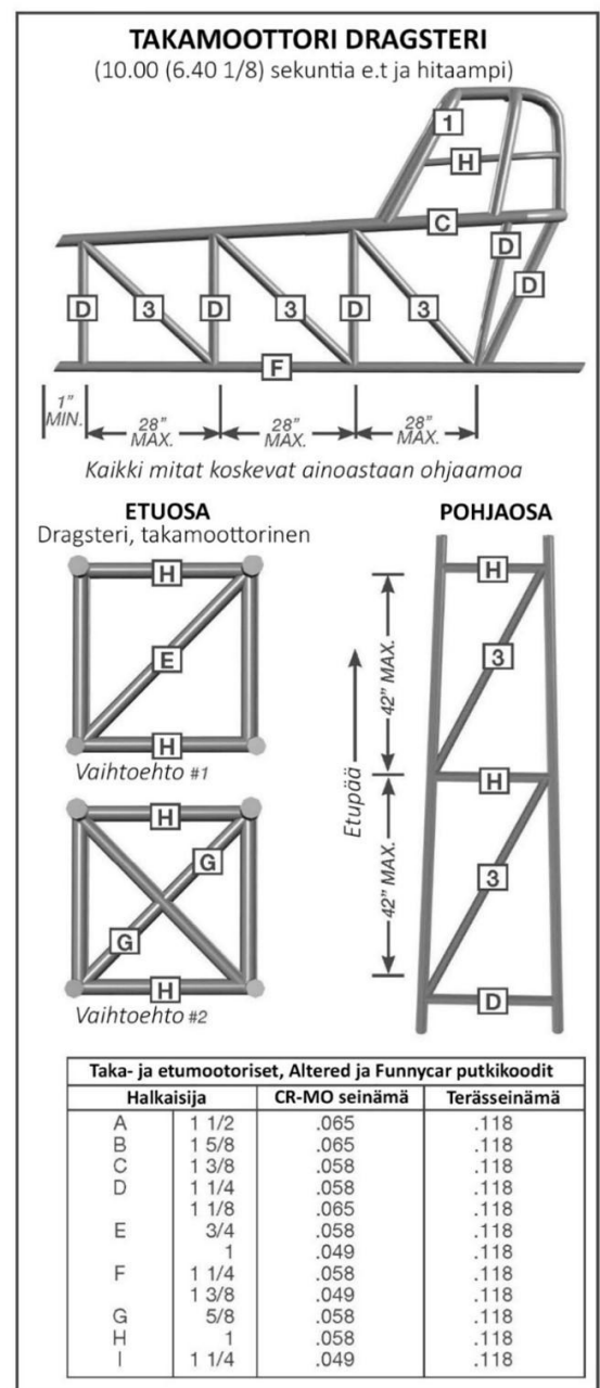
Kuva 15: Takamoottori dragsteri
