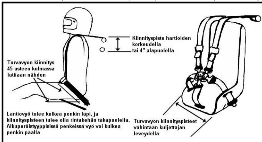
Kuva 23: Turvavyöt
